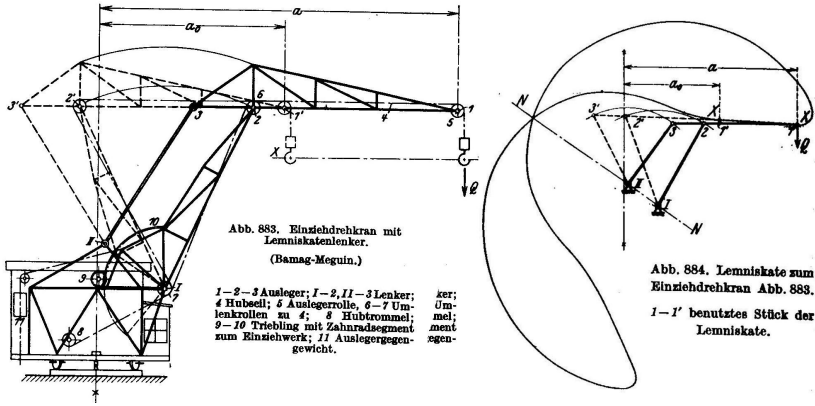
ABBILDUNG 10. Einziehrehkran mit Lemniska- tenlenker aus [17]
