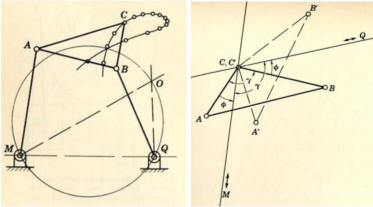
ABBILDUNG 7. Definition eines Pivotkreises und Beweissskizze (aus [16])
